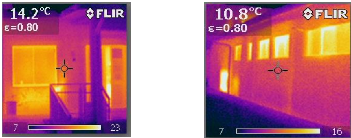
Figura 4.3 – Rilievo termografico della parete
